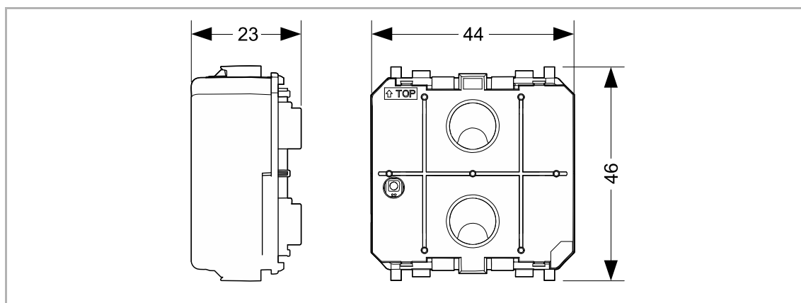
Fig. 3 : Dimensions (toutes les cotes en mm)
