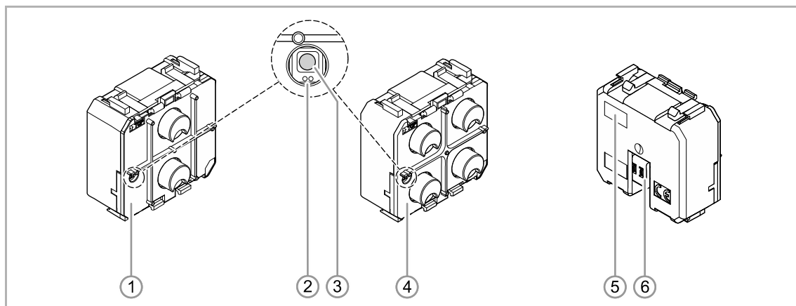
Afb. 2: Apparaatoverzicht schakelaar-aankoppelaars
