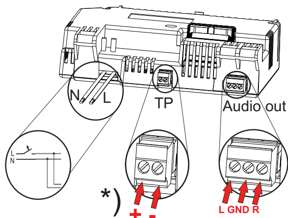
Fig. 17: Conexión eléctrica del módulo del bloque de alimentación
