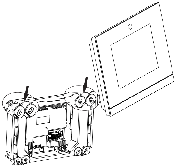
Fig. 20: Colocación de la pantalla en el marco de montaje
