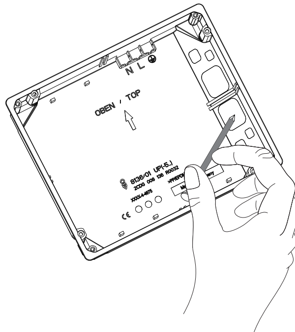
Fig. 10: Perforar la membrana de paso de cables
